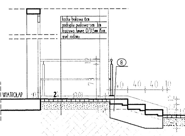
PRZEKROJ X9-X9 (wysokość stopnia - 12cm)
