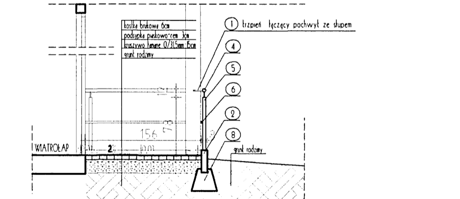
PRZEKROJ X3-X3
