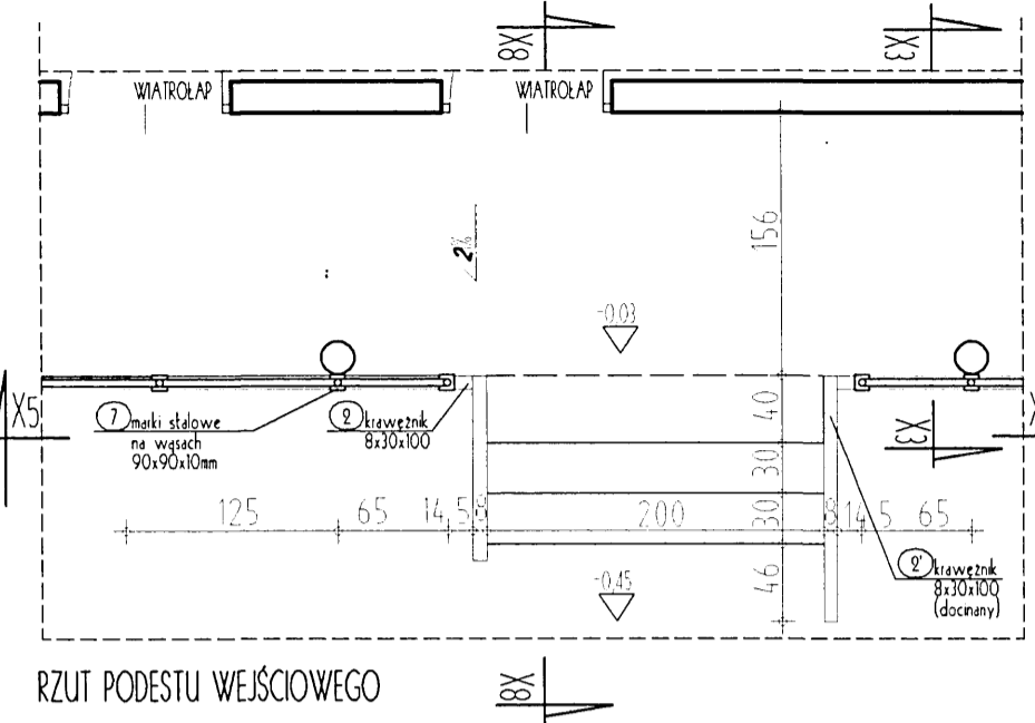
DETAL E - 4 szt.
