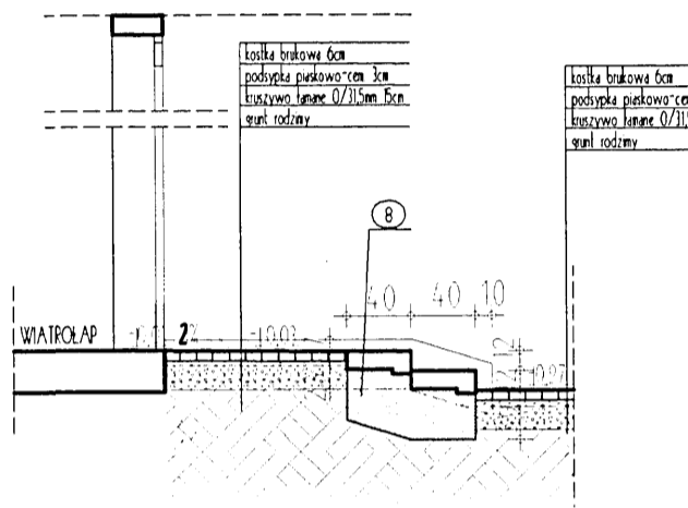
PRZEKROJ X12-X12 (wysokość stopnia - 12cm)
