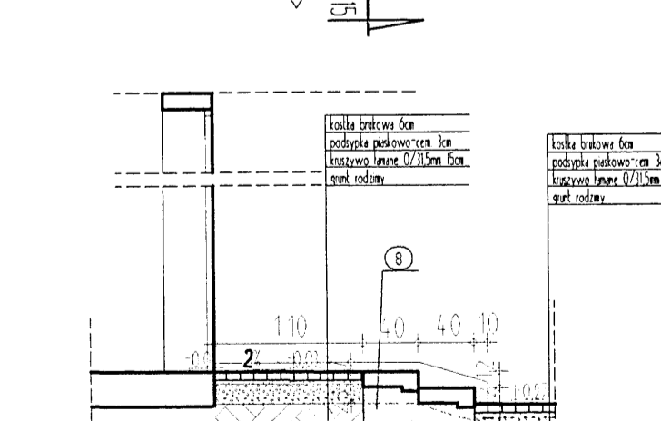
PRZEKROJ X15-X15 (wysokość stopnia - 12cm)
