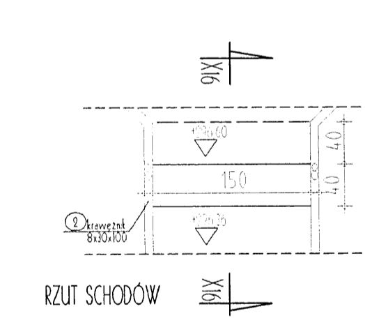
DETAL Ł - 1 szt.
