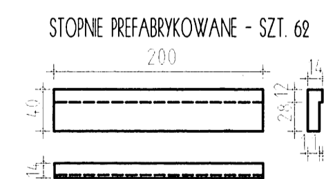
STOPNIE PREFABRYKOWANE - SZT. 62
