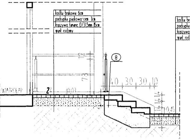
PRZEKROJ X8-X8 (wysokość stopnia - 14cm)
