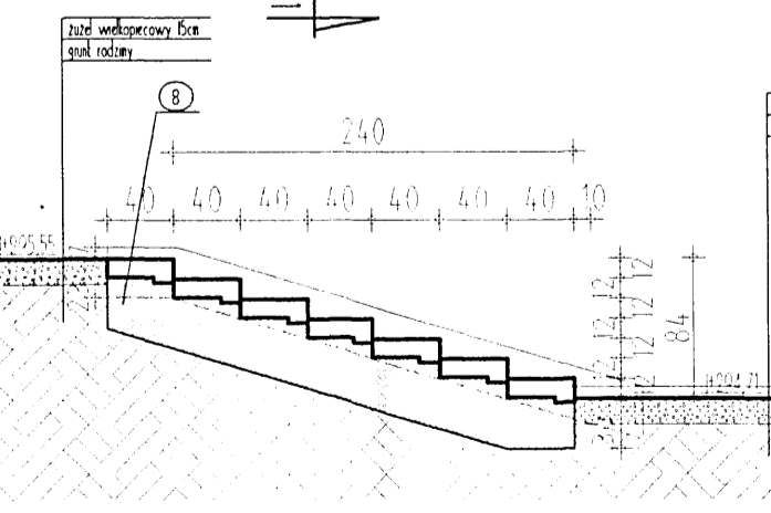
PRZEKROJ X11-X11 (wysokość stopnia - 12cm)
