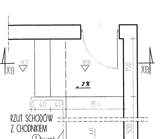
DETAL J - 1 szt.
