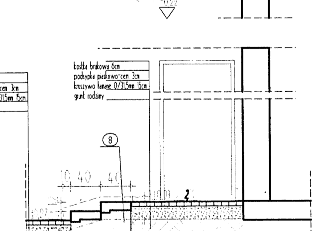
PRZEKROJ X13-X13 (wysokość stopnia - 12cm)
