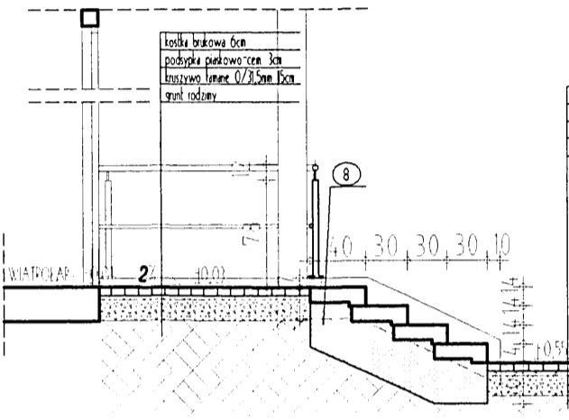
PRZEKROJ X10-X10 (wysokość stopnia - 14cm)
