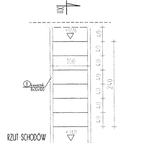
DETAL H - 1 szt.
