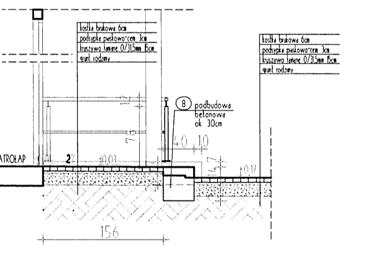
PRZEKROJ X4-X4 (wysokość stopnia - 14cm)
