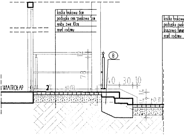
PRZEKROJ X6-X6 (wysokość stopnia - 14cm)
