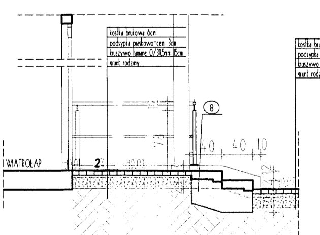
PRZEKROJ X7-X7 (wysokość stopnia - 12cm)
