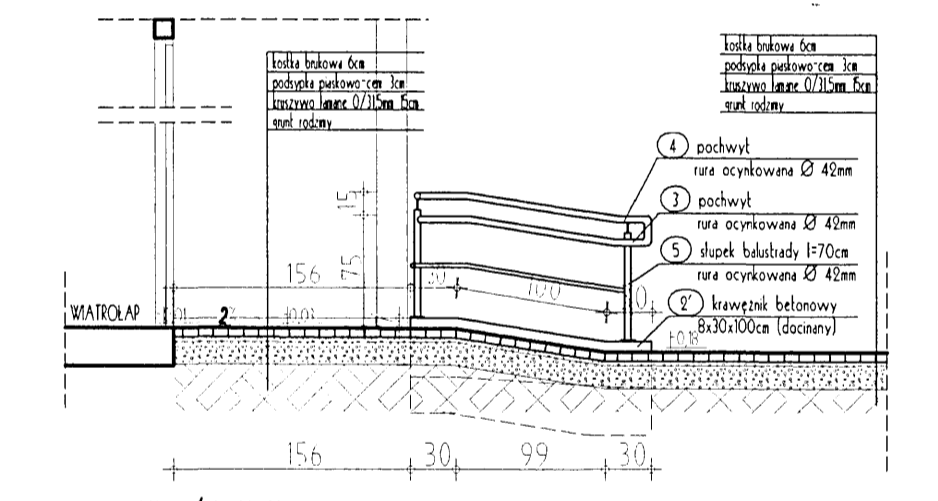
PRZEKROJ X1-X1
