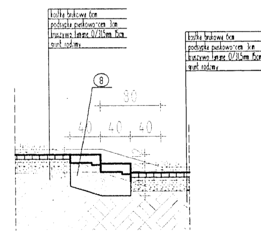
PRZEKROJ X16-X16 (wysokość stopnia - 12cm)
