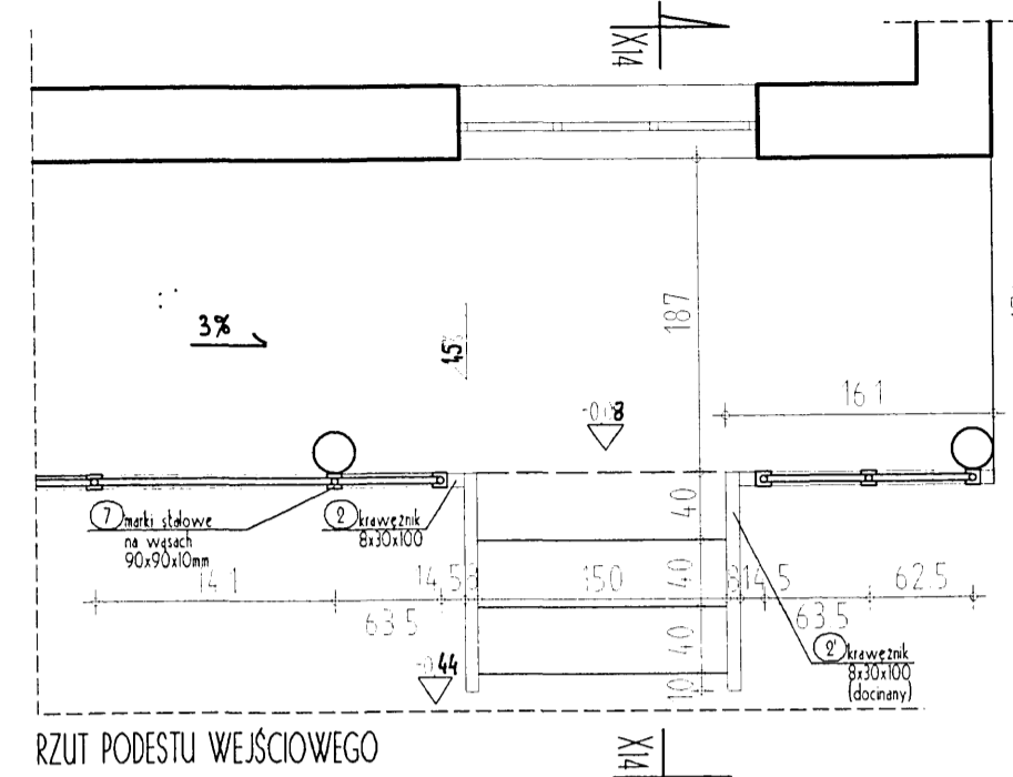
DETAL K - 1 szt.
