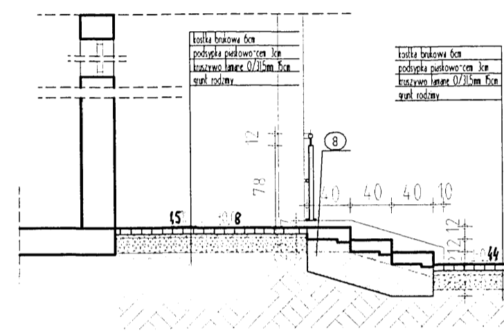
PRZEKROJ X14-X14 (wysokość stopnia - 12cm)
