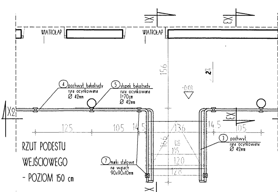
DETAL A - 4 szt.
